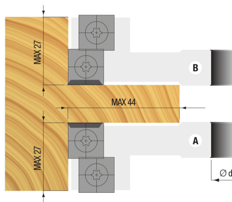
COMBINAZIONI POSSIBILI CUTTERHEAD COMBINATIONS FRÄSE-KOMBINATIONEN
